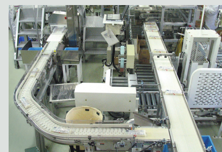
そうめん工場 1モーターで直線+カーブ+直線が駆動できる省エネ性が採用の決め手になりました
