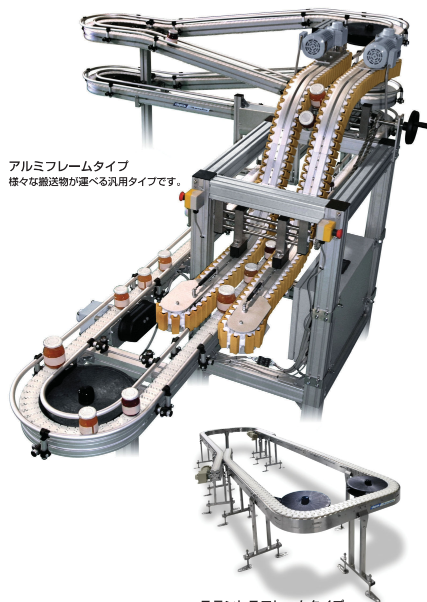
ステンレスフレームタイプ 洗浄や清掃が簡単なHACCP対応タイプです。
