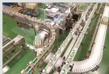
飲料工場 個装ラインと外装ラインの立体交差。搬送物の幅に合わせたチェーン幅をセレクトできます
