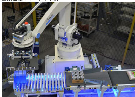
複数種類のワークの移載
