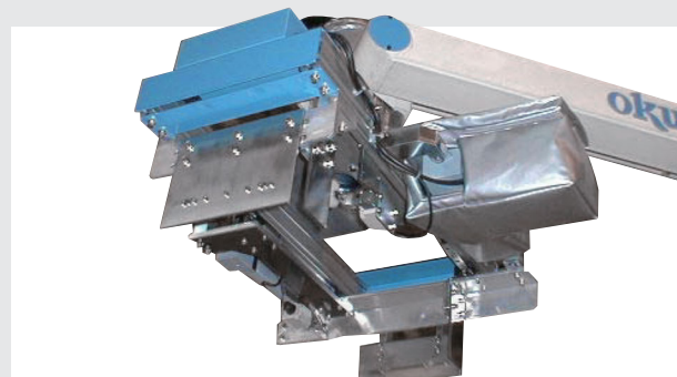
▲ハンドの開閉もモータで行う
